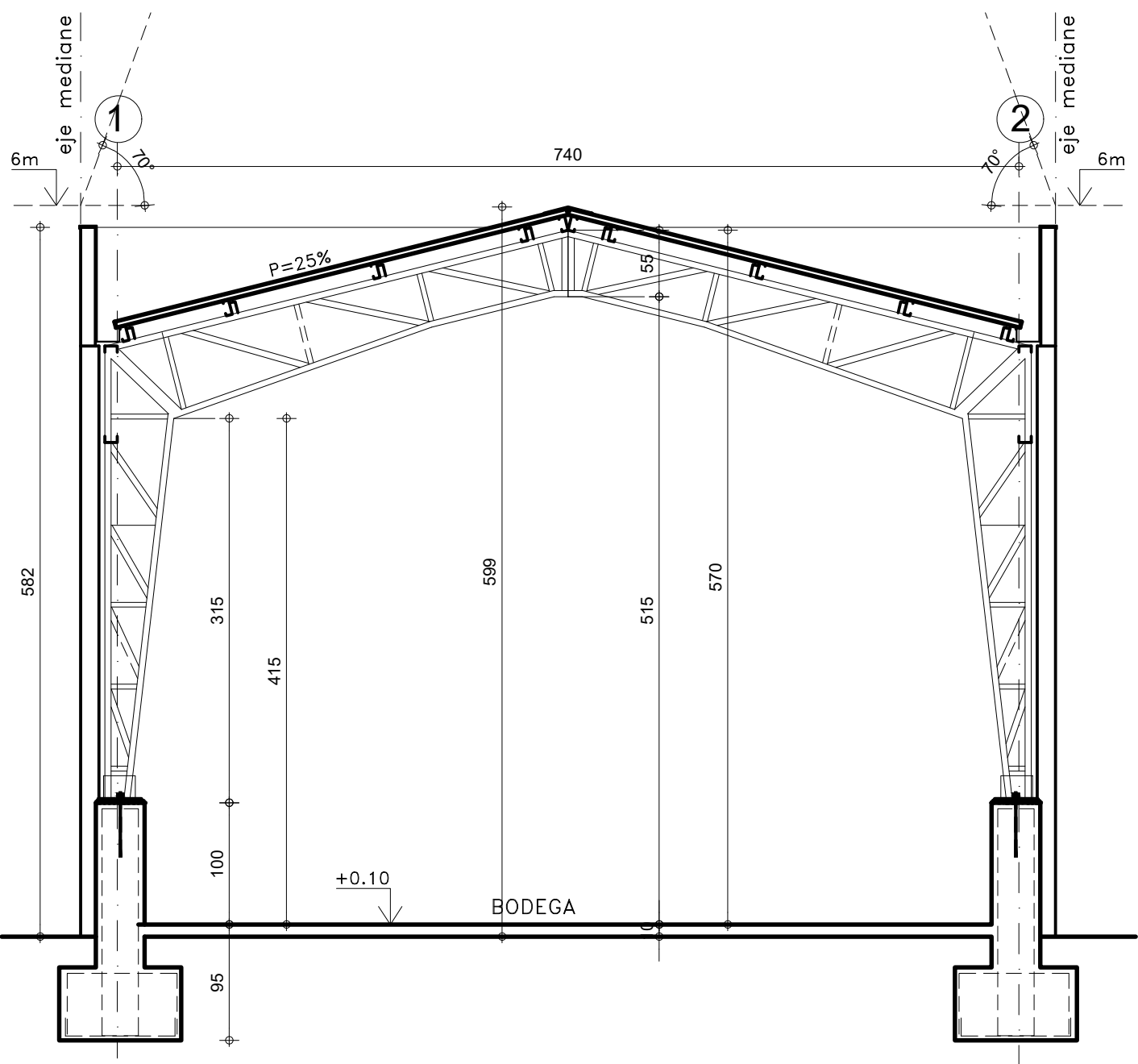
2 CORTE A-A 1:50
