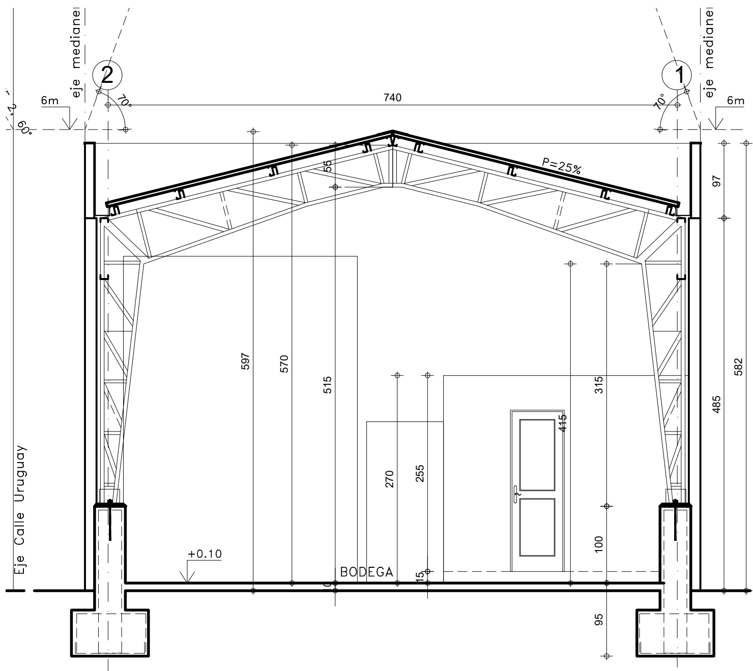
3 CORTE B-B 1:50
