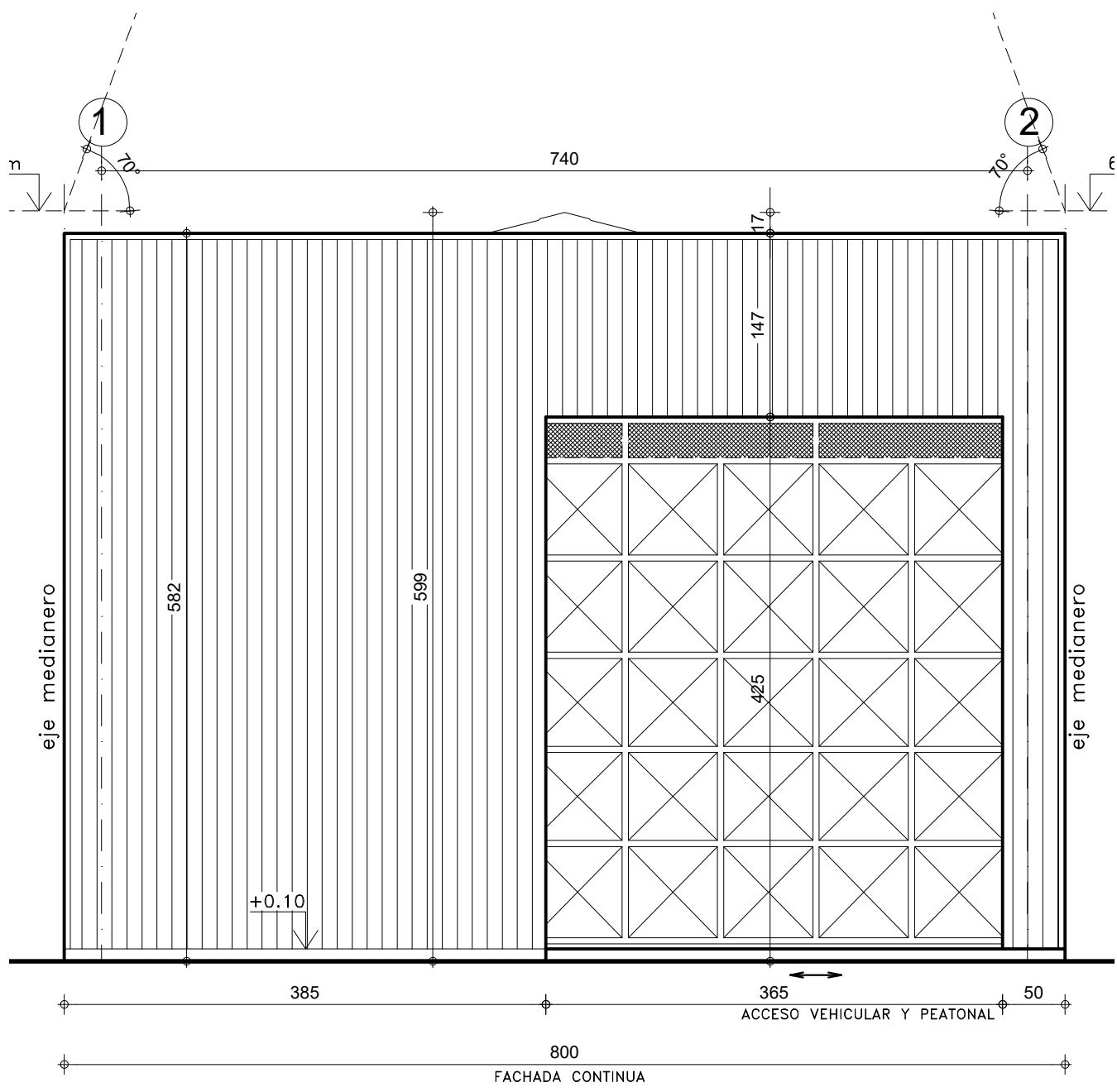
1 ELEVACION ORIENTE (CALLE URUGUAY) 1:50
