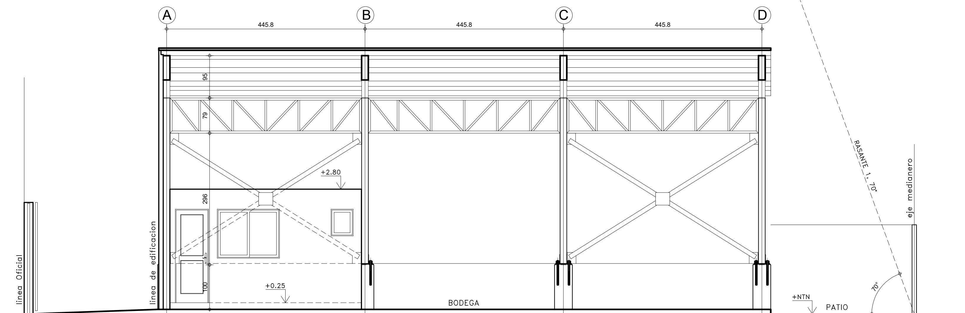
2 CORTE A-A 1:50
